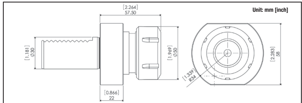
ER E4 DIN 6499
